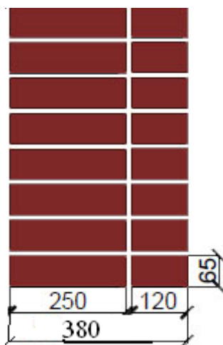
Ширина стены в 1,5 кирпича
